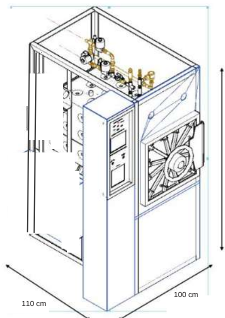
CAD vista isometrica
